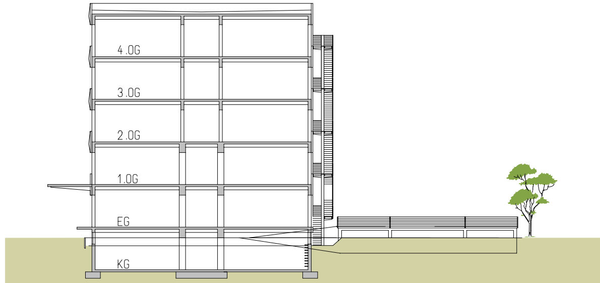
Schnitt Haus 11 A und Parkdeck I
